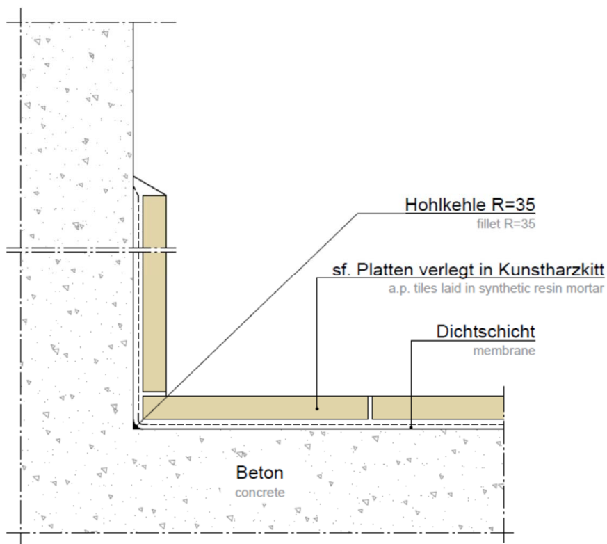
Abbildung 1: Boden-/Wandanschluss und Sockelausbildung
