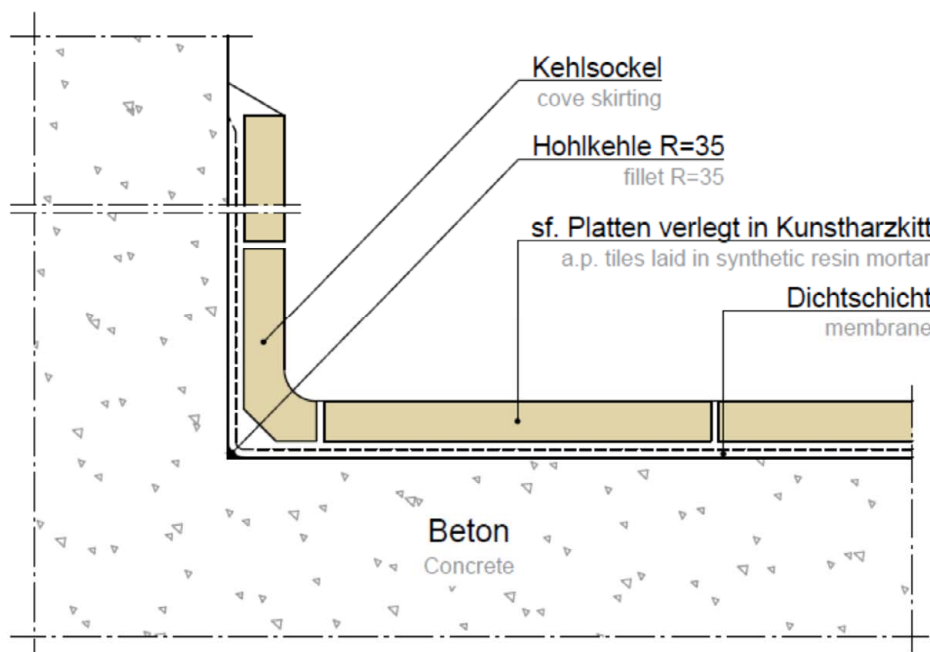
Abbildung 2: Boden-/Wandanschluss (Hohlkehle) und Sockelausbildung
