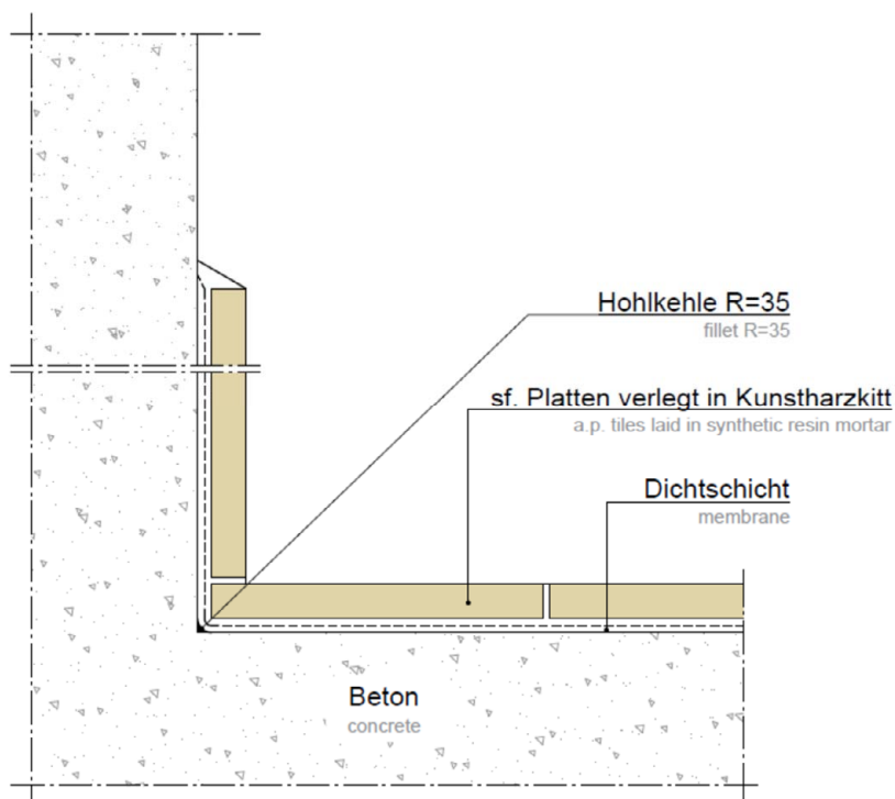
Abbildung 1: Boden-/Wandanschluss und Sockelausbildung
